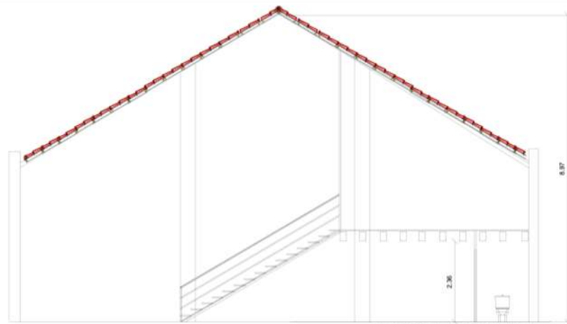
SECCION LONGITUDINAL REFORMADA Area total en altura 103.57 m 2 Volumen total taller 472.28 m 3
